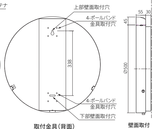
取付金具(背面)
